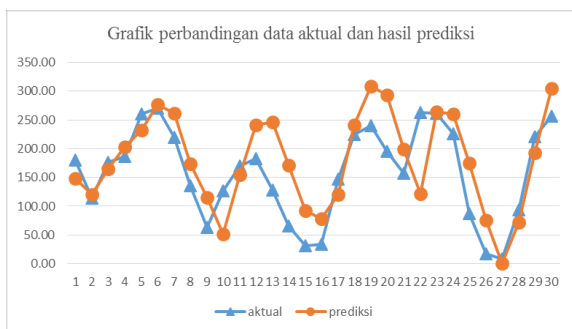
Gambar 6 Hasil prediksi M+1 dengan Generational Replacement
