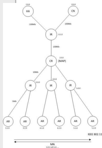
Gambar 2. Topologi jaringan
