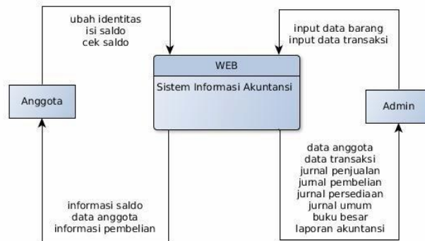
Gambar 4 Rancangan diagram konteks sistem
