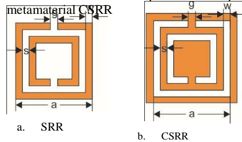
Gambar 3.7 Dimensi Struktur Metamaterial
