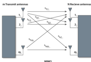
Gambar 2.4 Sistem MIMO [13]
