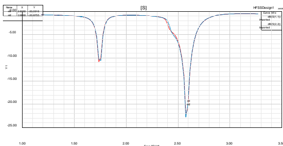
Gambar 3.15 Return Loss Antena MIMO Metamaterial dengan jarak dp = 52 mm
