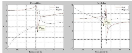
Gambar 3.11 Nilai permitivitas dan permeabilitas material
