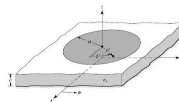
Gambar 2.1 Geometri antena mikrostrip patch lingkaran [7]
