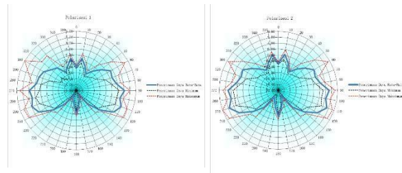
Gambar 4.7 Polarisasi antenna
