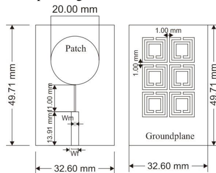
Gambar 3.12 Desain dan ukuran antena tunggal metamaterial
