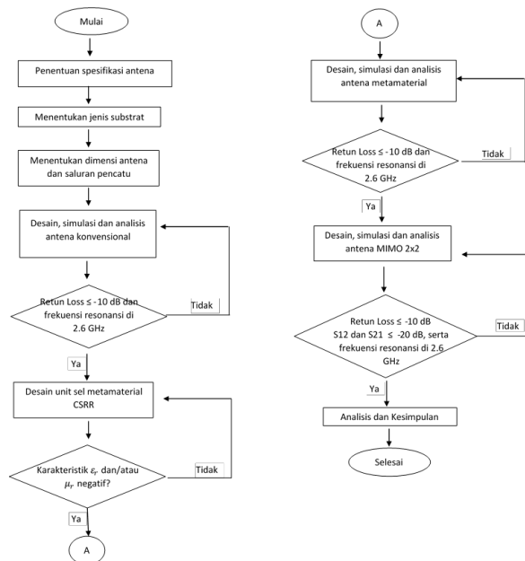
Gambar 3.1 Diagram alir perancangan antenna
