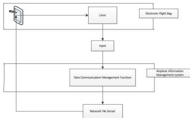
Gambar 3-2 Cara Kerja EFB
