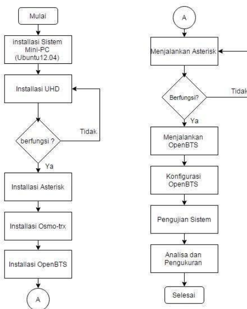
Gambar 3.1-2 Flowchart perancangan sistem.
