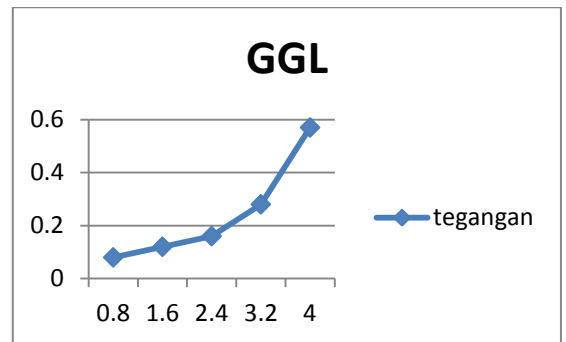
Gambar 4.2 Grafik GGL yang dihasilkan terhadap beban
