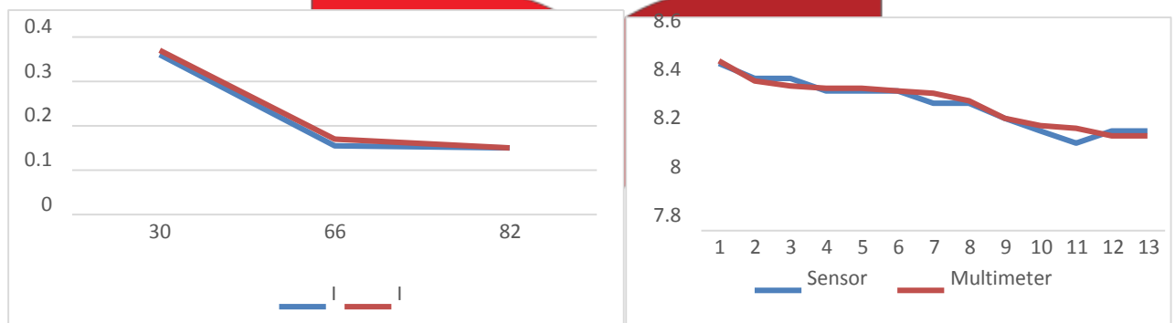
(a) Pengujian Sensor Arus dan (b) Pengujian Sensor Tegangan
