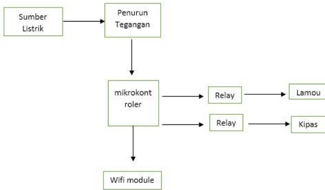
Gambar 3.2 Diagram blok perancangan
