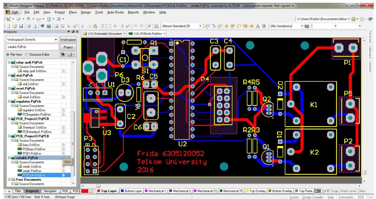
Gambar Skematik setelah di eksporse ke PCB
