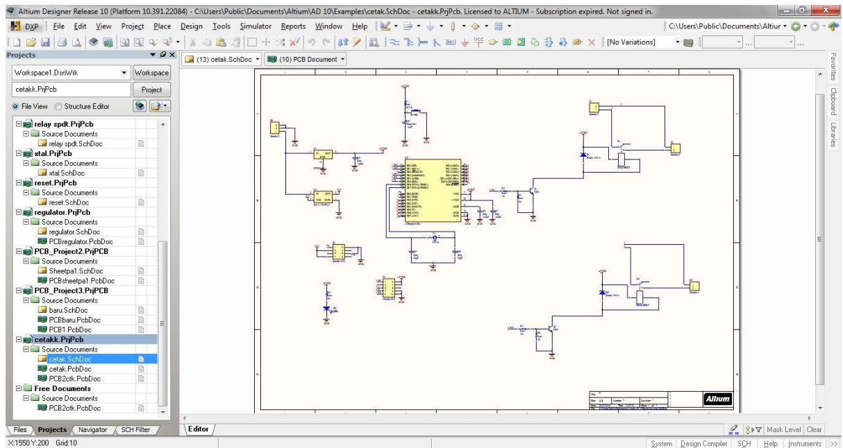
Gambar Skematik Sistem Minimum
