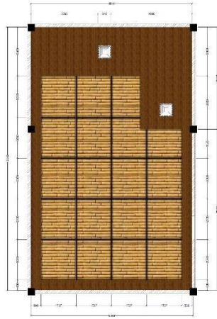
Gambar 3.5. Denah plafon & pengaplikasiannya pada ruang perawatan VVIP sumber: data pribadi
