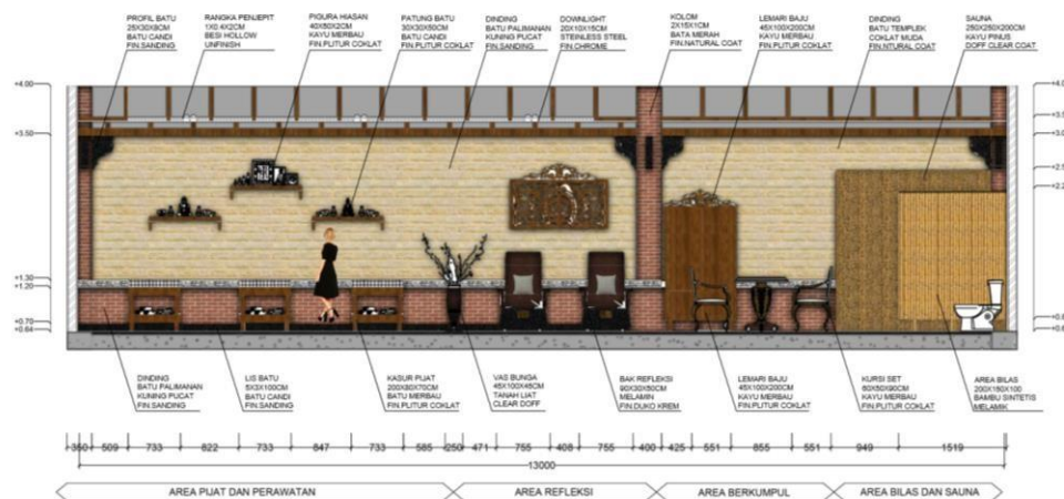
Gambar3.4. Tampak Potongan Ruang Perawatan VVIP
