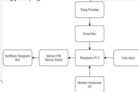
Gambar 3. 4 diagram blok perancangan
