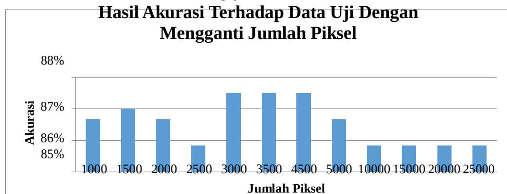
Gambar Grafik 4.2 Perhitungan Akurasi Terhadap Data Uji Dengan Mengganti Jumlah Piksel
