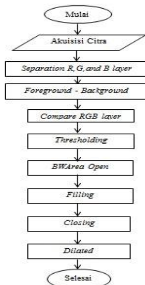
Gambar 3.1 Tahap Preprocessing
