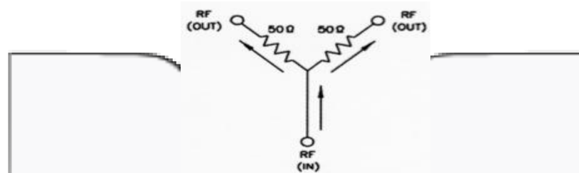
Gambar 2.1 Pembagi Daya
