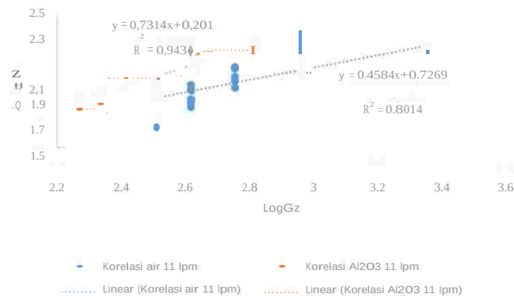
Gambar 4.4 Grafik perbandingan persamaan korelasi antara air dan nanofluida air- \text{Al}_2\text{O}_3
