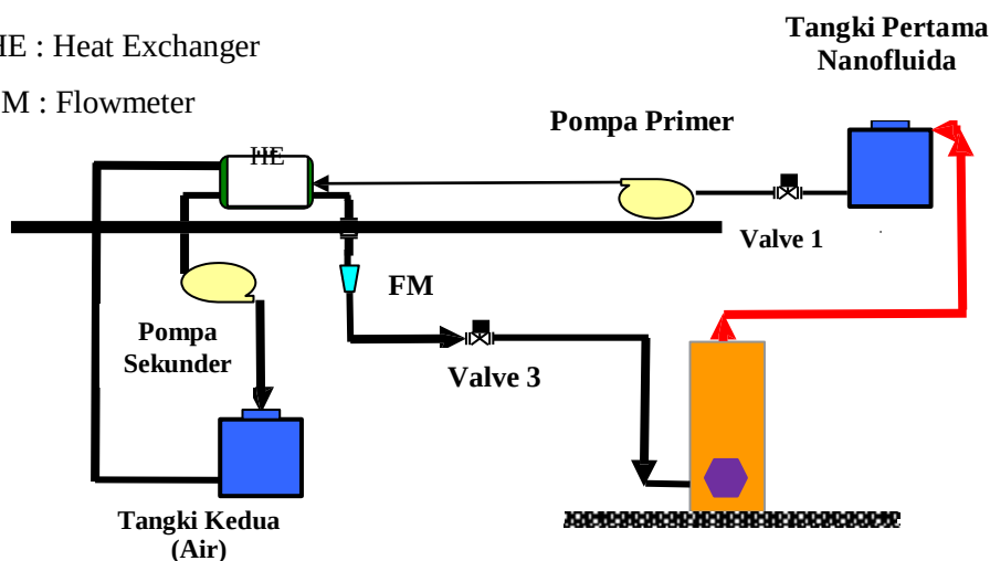
Gambar 2.3 Rangkaian alat uji
