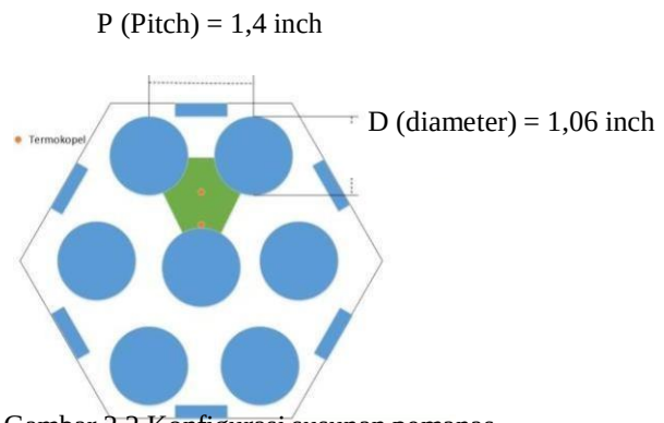
Gambar 2.2 Konfigurasi susunan pemanas
