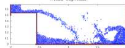
Gambar 13 Simulasi air terjun ketinggian 0,55 meter
