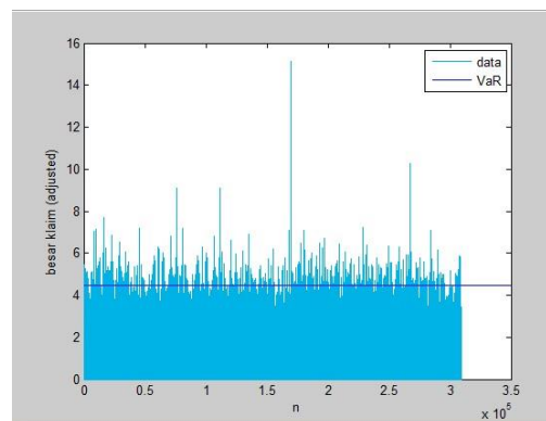
Gambar 7 Grafik Data Frekuensi Terhadap Nilai Dengan VaR 95%
