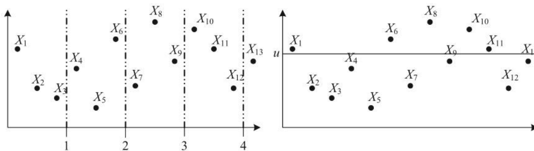
Gambar 2.1 Metode BM (kiri) dan Metode POT (kanan)
