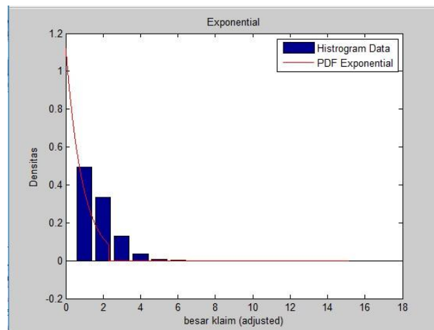
Gambar 2 Curve Fitting distribusi mixture exponential dengan satu lambda.
