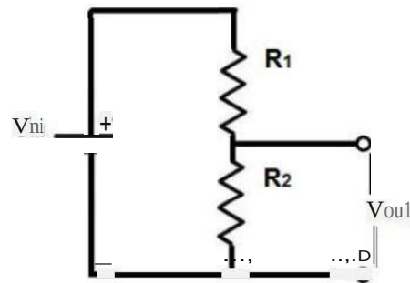
Gambar 4. Sensor Tegangan
