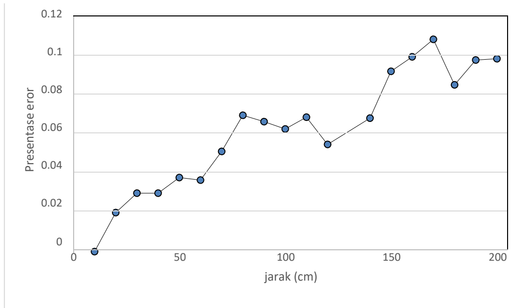
Gambar 5. Grafik presentase error terhadap jarak pada pengujian sensor ultrasonik
