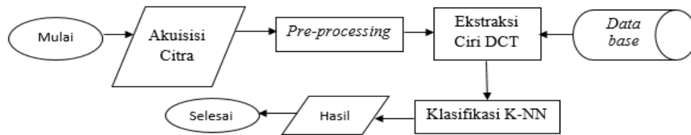
Gambar 3. 3 Diagram Alir Proses Identifikasi Tahap Citra Uji
