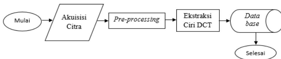
Gambar 3. 2 Diagram Alir Proses Identifikasi Tahap Citra Latih
