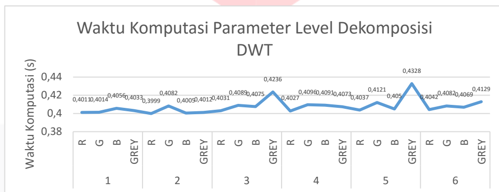
Gambar 4.3 Waktu Komputasi Level Dekomposisi DWT
