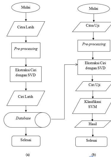
Gambar 3.3 Diagram alir proses latih dan uji
