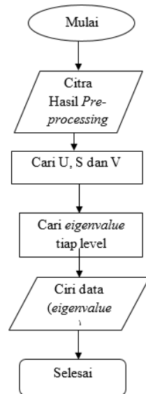
Gambar 3.2 Diagram Alir Ekstraksi Ciri SVD
