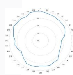
Gambar 4.4 Polarisasi
