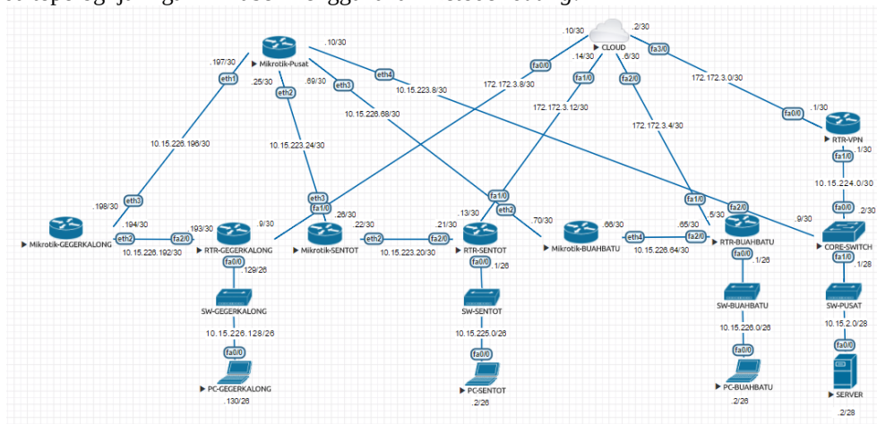
Gambar 12 Topologi simulasi jaringan nirkabel usulan metode routing
