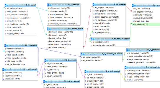
Gambar 3.11 Skema Relasi
