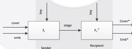
Gambar 2.1 Sistem Steganografi
