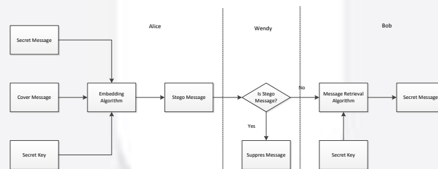
Gambar 2.2 Proses steganalisis secara umum
