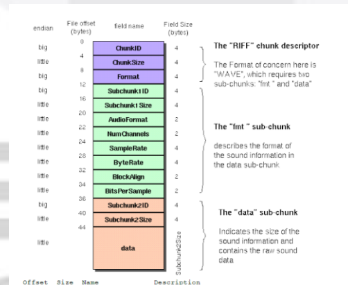
Gambar 2.3 Bagian Struktur file .WAV [6]
