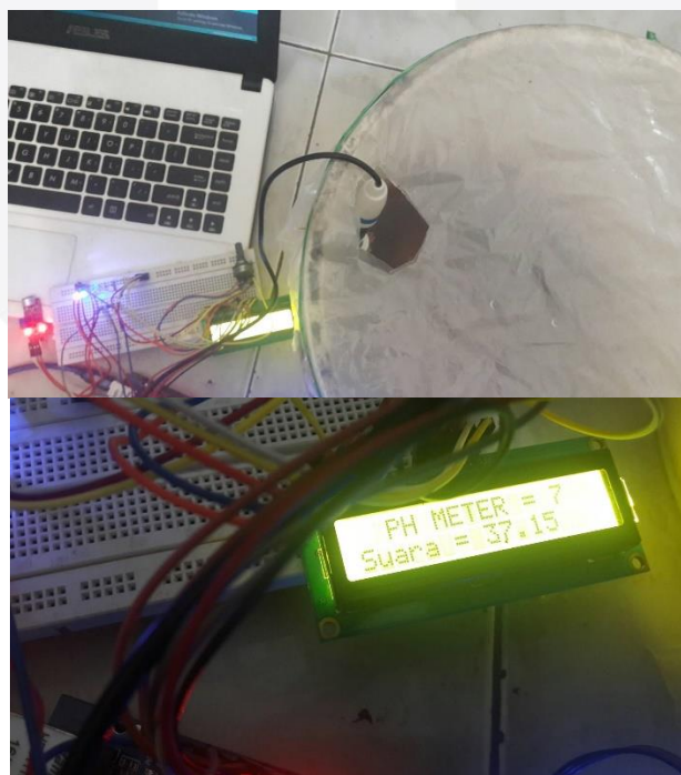
Gambar 8 Pengujian mengukur tingkat pH pada air yang berisi ikan lele
