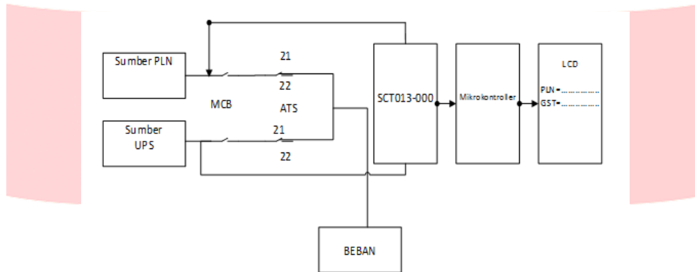
Gambar 1 Skema Pengujian Sensor Arus SCT013-000
