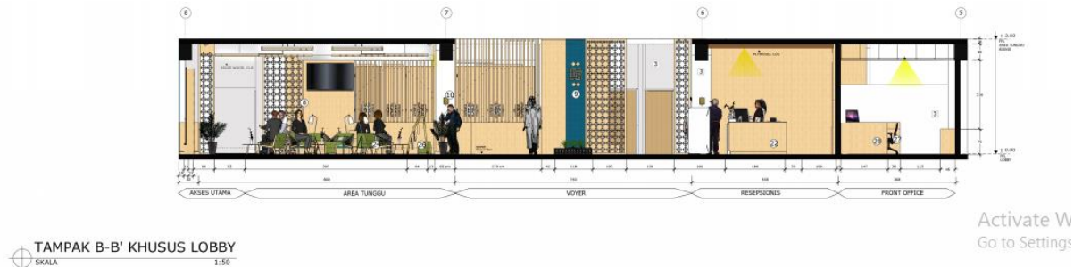
Gambar 4.3 Tampak Khusus Lobby
