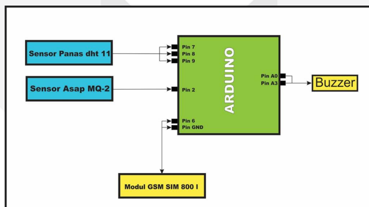
Gambar 3.2 Diagram blok sistem
