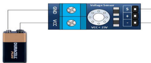
Gambar 3.3 Konfigurasi Sensor tegangan
