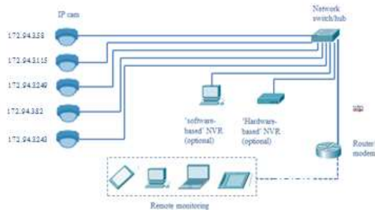
Gambar 3.2 Topologi sistem
