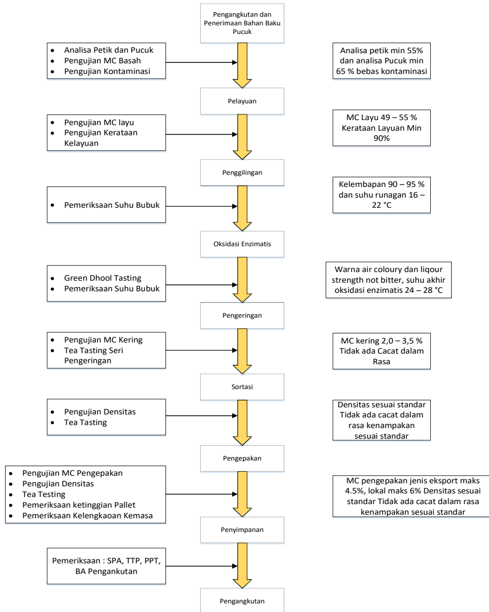
Gambar I.1 Alur Proses Produksi Bubuk Teh Hitam Orthodox
