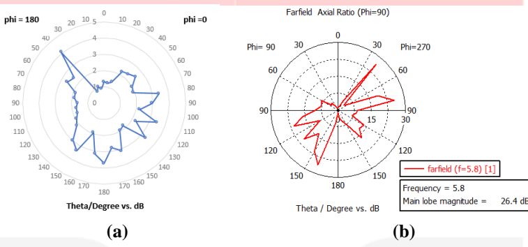
Gambar 10 Beamwidth Rasio Aksial elevasi antenna (a) Realisasi (b) Simulasi
