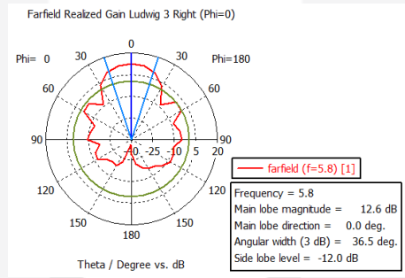
Gambar 11 Gain polarisasi sirkular RHCP antenna realisasi
