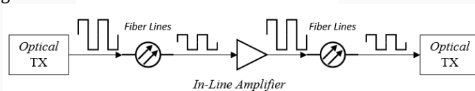
Gambar 2.2 Konfigurasi In-Line Amplifier
