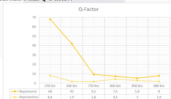
Gambar 4. 4 Hasil Simulasi Berdasarkan Nilai Q-Factor
