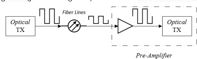
Gambar 2.3 Konfigurasi Pre-Amplifier
