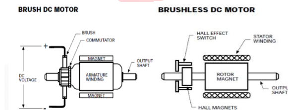
Gambar II-2 Kontruksi motor DC brush dan brushless
