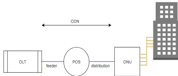
Gambar 2.3 Arsitektur FTTB
