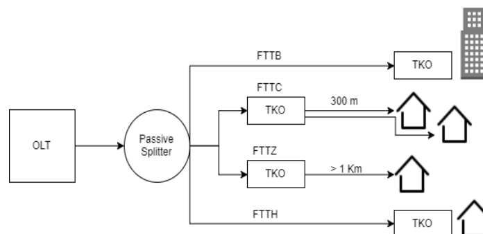
Gambar 2.2 Titik Konversi Optik FTTx
