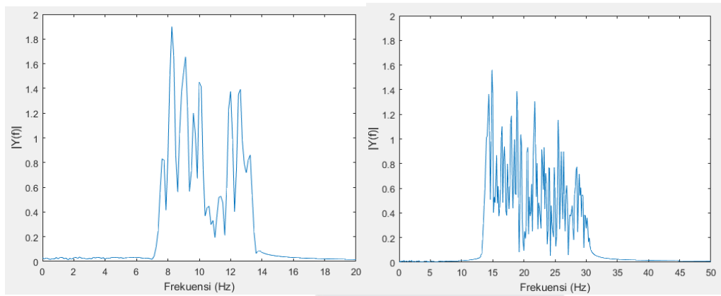
(a) (b) Gambar 4. 9 Hasil FFT sinyal (a) alfa dan (b) beta rumus
