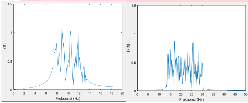
(a) (b) Gambar 4. 8 Hasil FFT sinyal (a) alfa dan (b) beta nama
