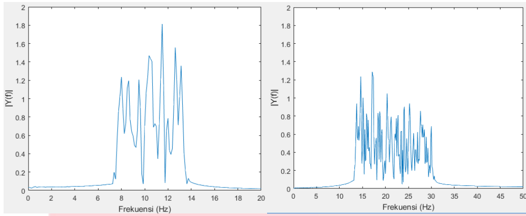
(a) (b) Gambar 4. 7 Hasil FFT sinyal (a) alfa dan (b) beta Alquran
