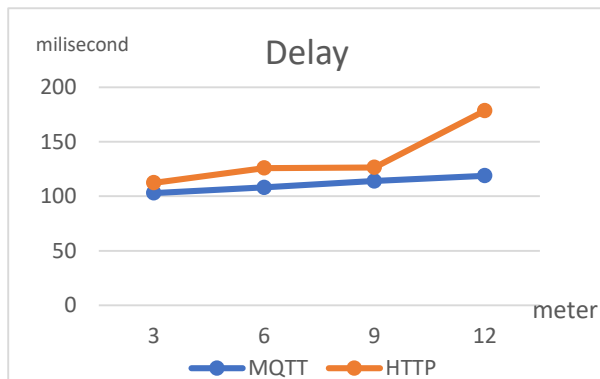
Gambar 4.1 Delay Terhadap jarak
