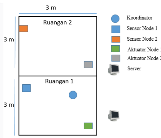
Gambar 3.6 Denah Pemasangan Sistem
