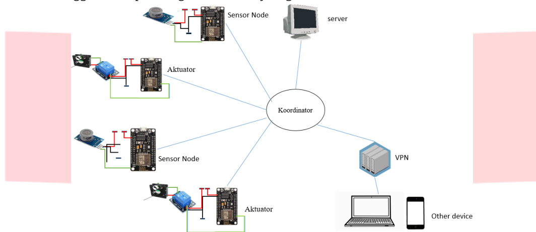
Gambar 3.5 Rancangan Keseluruhan Sistem
