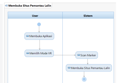
Gambar 9 Activity Diagram membuka Situs Pemantau Lalin
