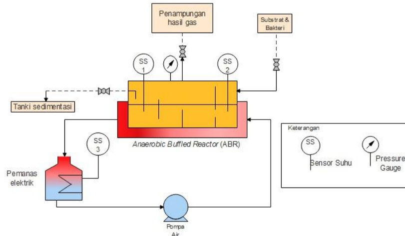
Gambar 2.3 Pengkondisian suhu pada substrat
