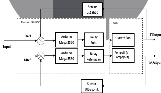
Gambar 3.1 Diagram Blok Sistem Secara Umum
