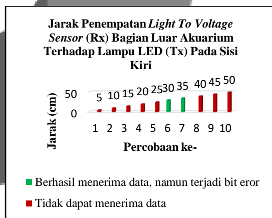
Gambar 4.18 Jarak Rx Di Sisi Kiri Aquarium Pada Ruangan Gelap (UVLC)
