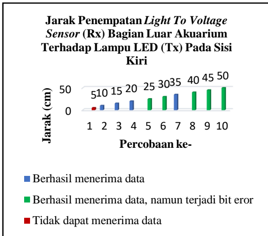
Gambar 4.6 Jarak Rx Di Sisi Kiri Aquarium Pada Ruang Terang (VLC)
