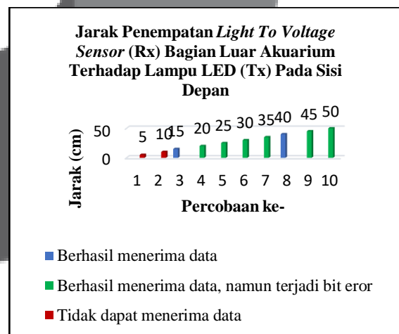
Gambar 4.5 Jarak Rx Di Sisi Depan Akuarium Pada Ruangan Gelap (VLC)
