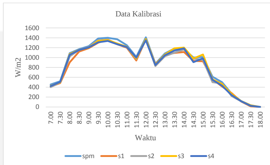
Gambar 3.1 Data Kalibrasi
