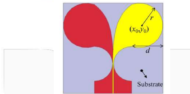
Gambar 1. Bentuk konfigurasi Antena Vivaldi antipodal sirkular
