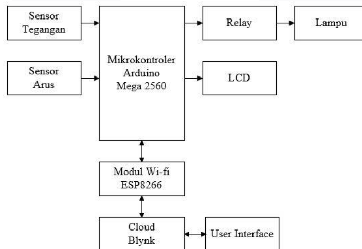
Gambar 3.2. Diagram Blok Integrasi Perangkat IoT
