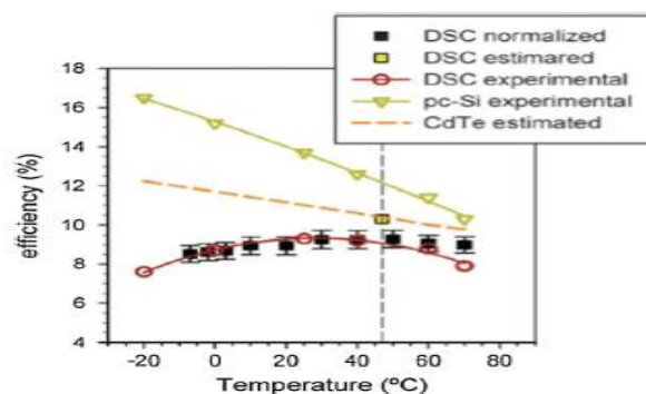
Gambar 4.2 Grafik efisiensi listrik terhadap suhu panel surya [15]
