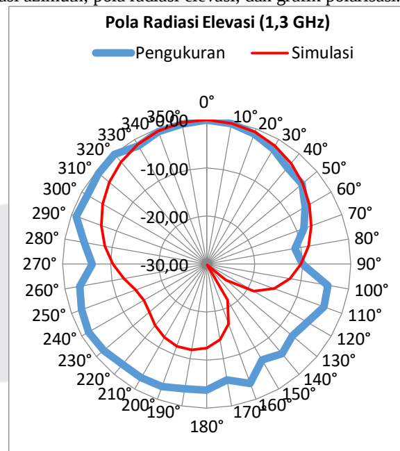
Gambar 13. Grafik Pola Radiasi Elevasi
