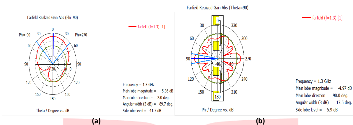
Gambar 7. Pola Radiasi (a) Arah Azimuth dan (b) Arah Elevasi
