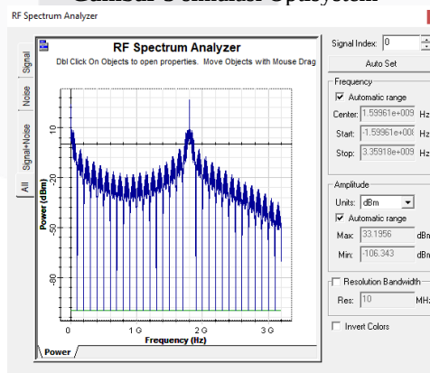
Gambar 6 Hasil RF Analyzer sebelum di modulasi
