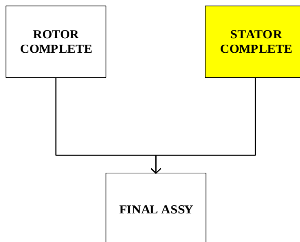
Gambar I. 3 Precedence Diagram Secara Umum Motor Listrik BLDC 5 kW
