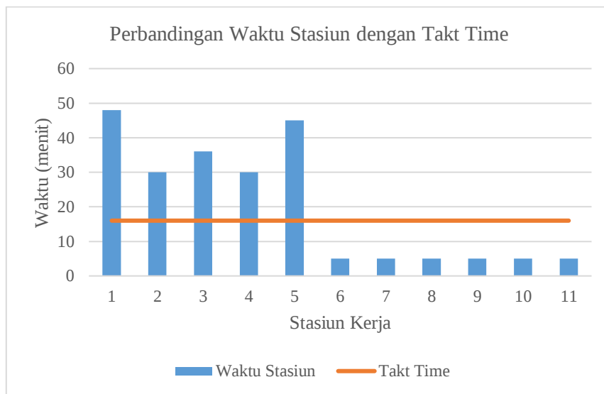
Gambar I. 4 Perbandingan Waktu Stasiun dengan Takt Time
