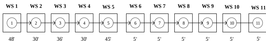
Gambar I. 5 Lintasan Perakitan Aktual Sub-Assembly Stator Complete
