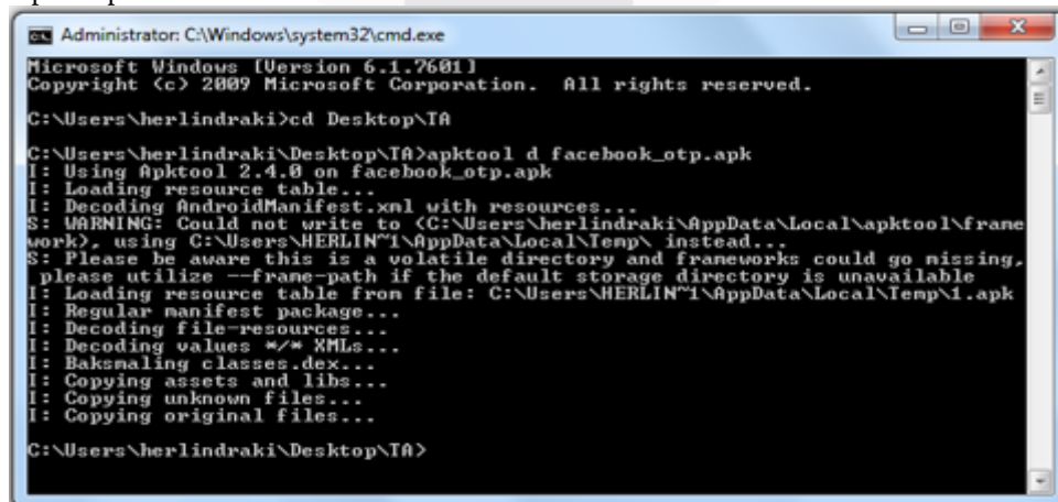
Gambar 3 penggunaan apktool
