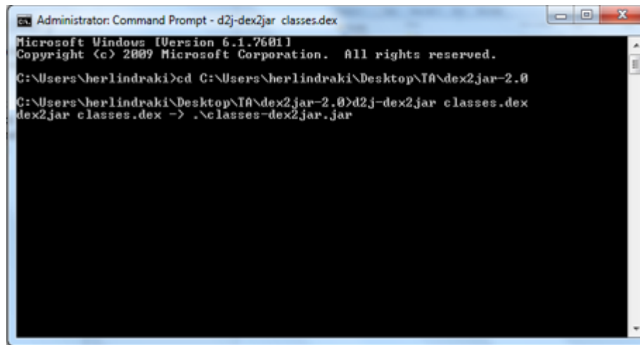
Gambar 1 Menggunakan dex2jar
